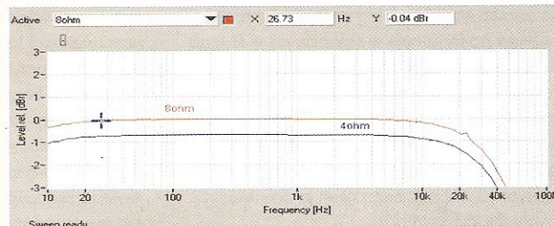
Rys. 1. Pasma przenoszenia
