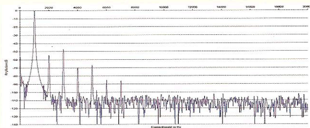
Rys. 2. Zniekształcenia harmoniczne
